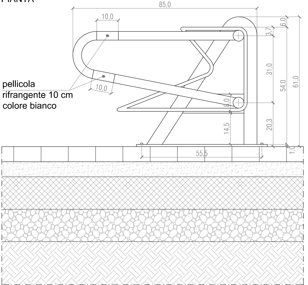
VISTA LATERALE
