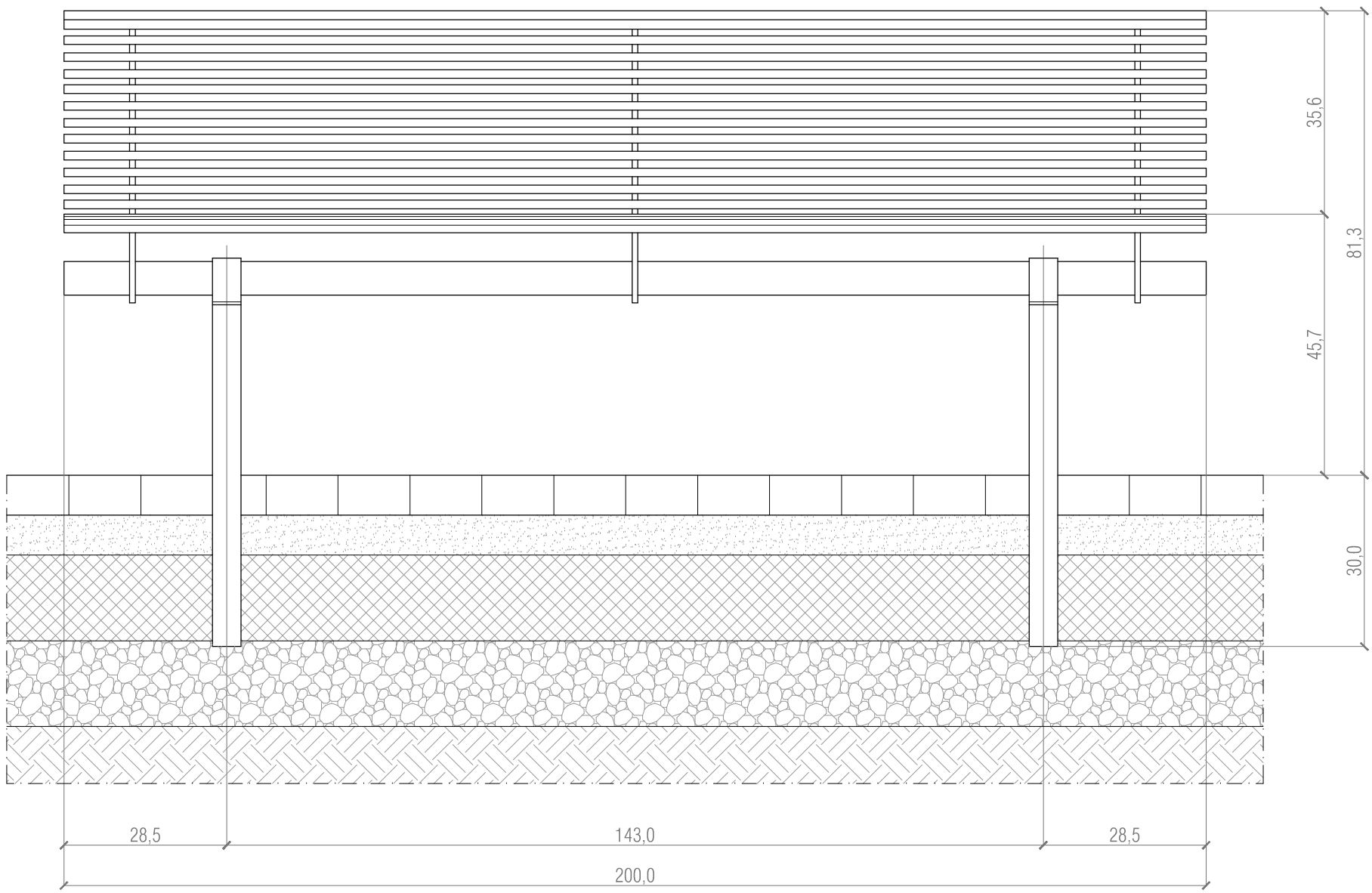
VISTA FRONTALE
