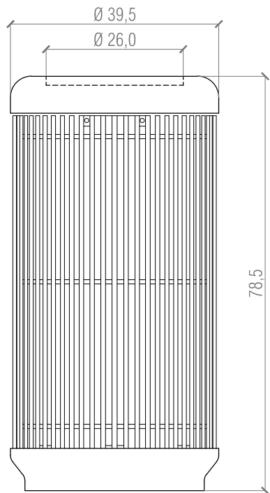
VISTA FRONTALE
